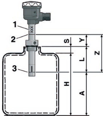
Bild 12: Standaufnehmer einstellen
